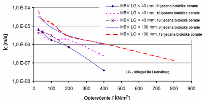
Slika 3. Ovisnost koeficijenta propusnosti o efektivnim naprezanjima [7]
