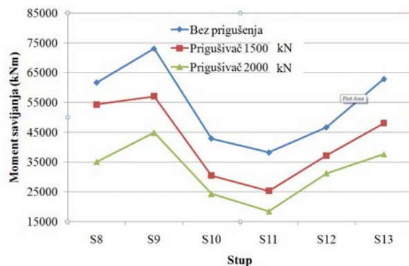
Slika 16. Momenti savijanja u stupovima za neprigušenu i prigušenu konstrukciju
