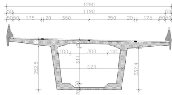
Slika 12. Poprečni presjek između stupova
