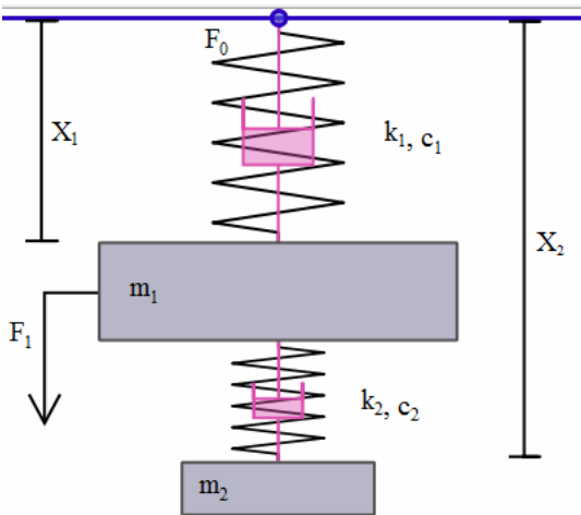
Slika 8. Mehanička shema uređaja s usklađenom masom
