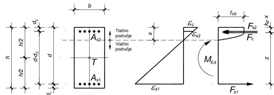
Slika 4. Pravokutni presjek naprezan momentom savijanja
