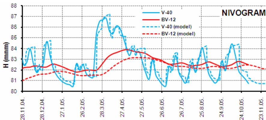
Slika 6. Usporedba izmjerenih i izračunanih nivograma za piezometre na pozicijama V-40 (crpna stanica hidročvora Sava) i BV-12 (Velika Kapanica) tijekom analiziranoga baždarnog razdoblja od 28.11.04. do 28.11.05.
