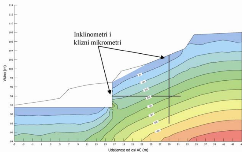
Slika 5. Pozicije ugrađene mjerne opreme na stac. 2 + 380
