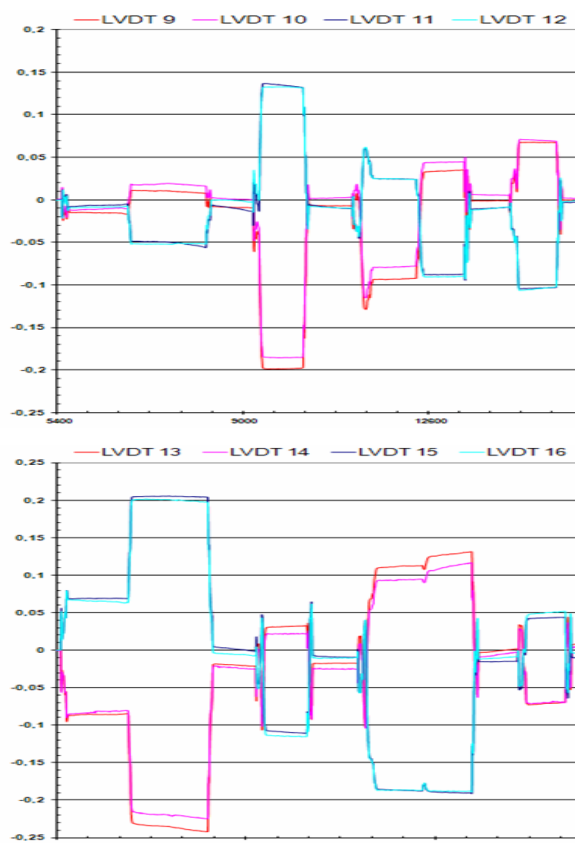
Slika 15. Vremenski tijek deformacija luka u presjecima 4-4 i 5-5
