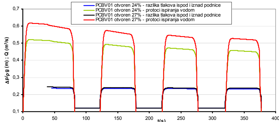
Slika 6. Prikaz vremenske varijacije protoka i razlika tlakova ispod i iznad podnice za otvorenosti regulacijskog ventila od 24 % (21,60 → ξPCBV01 = 100) i 27 % (24,30 → ξPCBV01 = 75)
