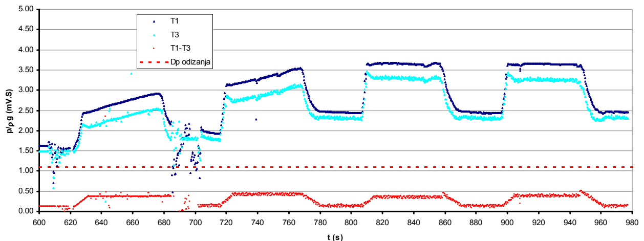
Slika 8. Prikaz vremenske serije izmjerenih tlakova u prvih četiri pulsa ispiranja vodom (mjerjenje u naravi – prema optimiziranom tehnološkom procesu)
