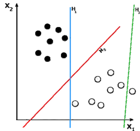
Slika 1. Primjeri razdvajajućih pravaca
