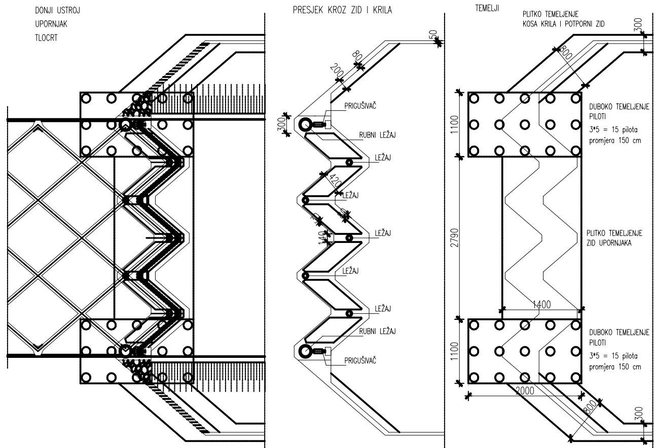
Slika 9. Upornjak mosta Bundeck
