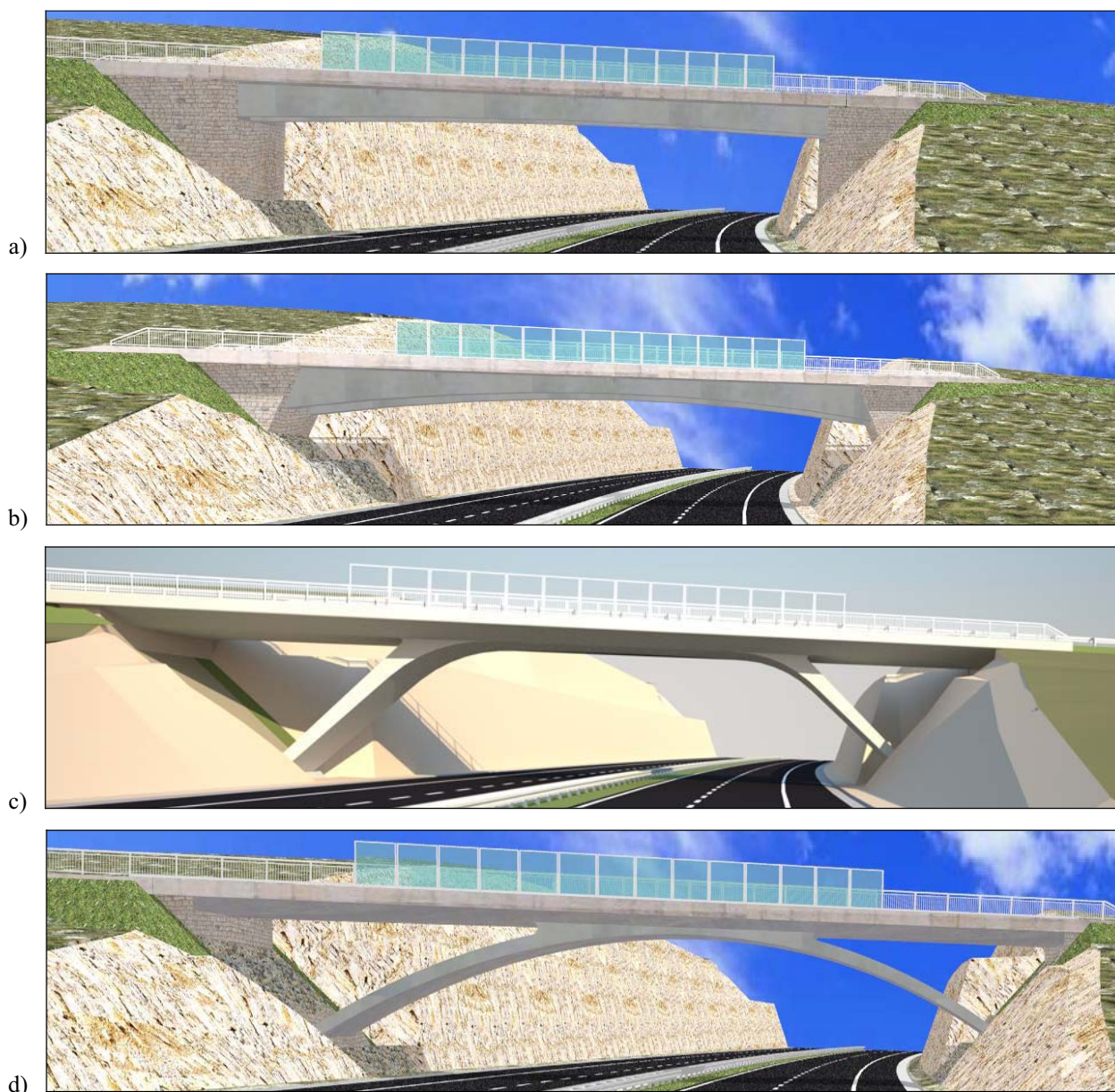
Slika 11. Nadvožnjak od betona velike čvrstoće: a) inačica 1, b) inačica 2, c) inačica 3 i d) inačica 4
