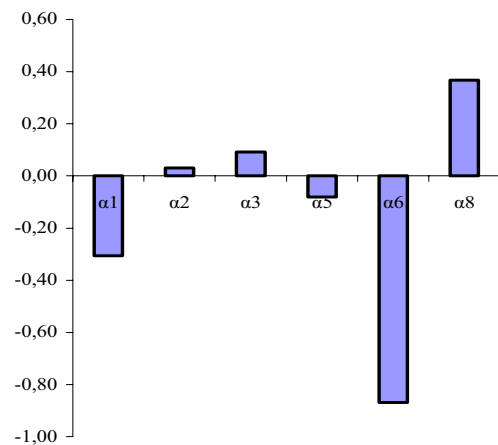
Slika 3. Faktori osjetljivosti (progib)
