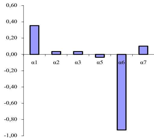
Slika 2. Faktori osjetljivosti (posmik)
