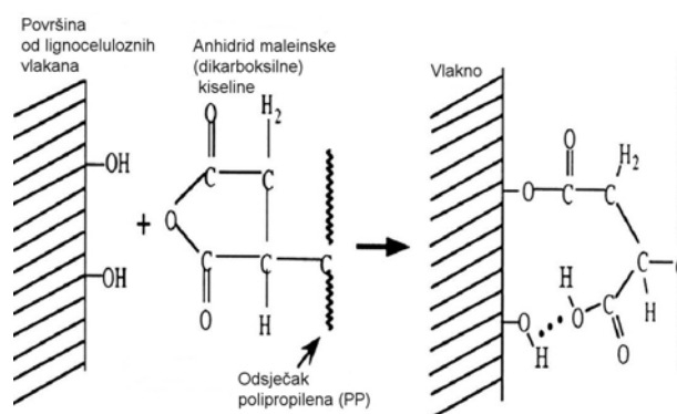
Slika 2. Formiranje estera
