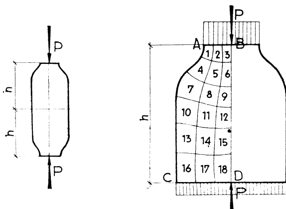
Slika 1. Trajektorije naprezanja koje je skicirao profesor Werner [4]
