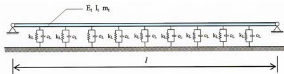
Slika 3. Matematički model kolosijeka (tračnica i ležaji)
