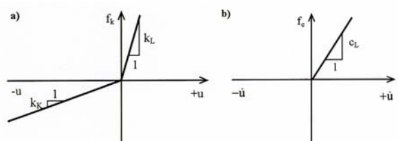
Slika 4. Model ponašanja ležaja: a) krutosti, b) prigušenje
