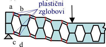
(c) Deformacija Vierendeelova nosača
