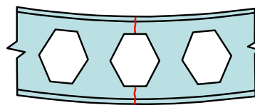
Slika 3. Otkazivanje saćastog nosača za poprečne presjeka s otvorom u hrptu
