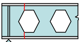
Slika 3. Otkazivanje saćastog nosača za poprečne presjeka s otvorom u hrptu
