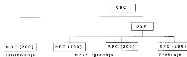
Slika 3. Shema inovativnih cementacijskih materijala i proizvodnih procesa; u zgradama su čvrstoće (vlačna za MDF, tlačna za HPC i RPC)
