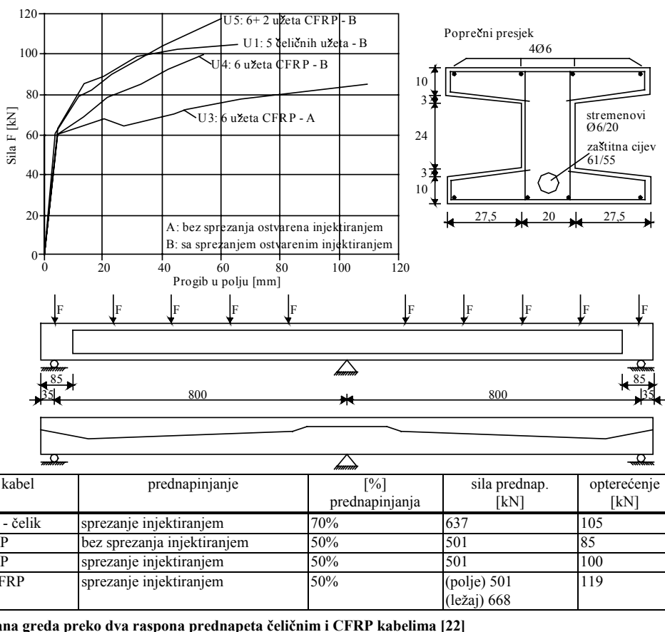
Slika 6. Kontinuirana greda preko dva raspana prednapeta čeličnim i CFRP kabelima [22]
