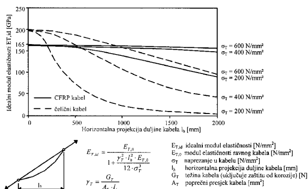
Slika 1. Idealni modul elastičnosti E T, id vješaljka (zatege) od čelika ili CFRP-a ovisno o horizontalnom rasponu zatege [20]
