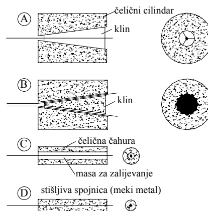
Slika 3. Sustavi sidrenja kabela (A i B – čelik, C i D – CFRP)
