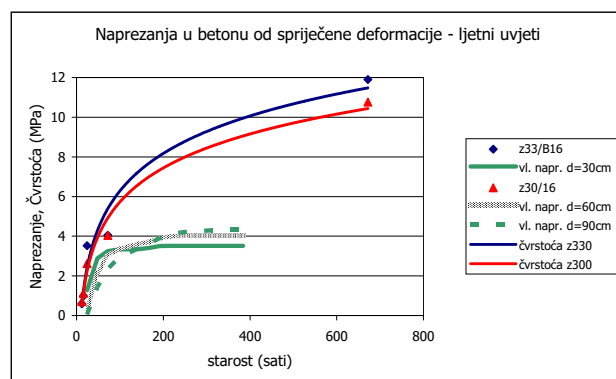
Slika 7. Prirast čvrstoće i naprezanja u betonu od spriječene deformacije za a) ljetne uvjete i b) zimske uvjete
