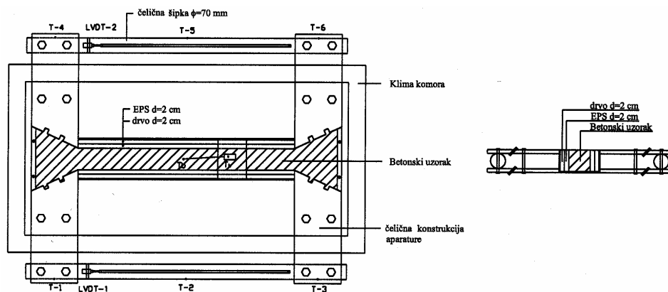
Slika 2. Shema konstrukcije aparature za mjerenje temperature i naprezanja u betonu
