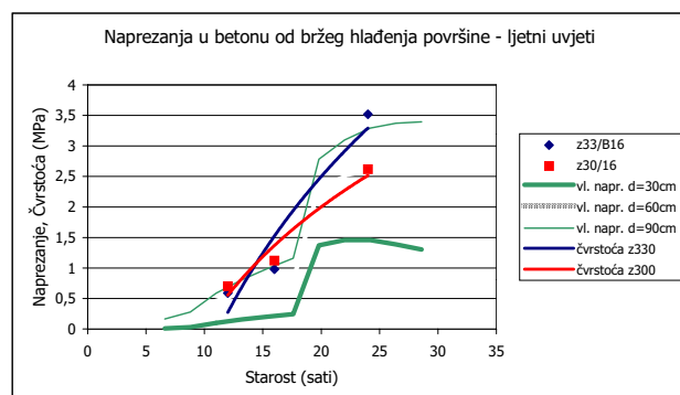
Slika 6. Prirast čvrstoće i naprezanja u betonu od brzog hlađenja površine za a) ljetne uvjete i b) zimske uvjete
