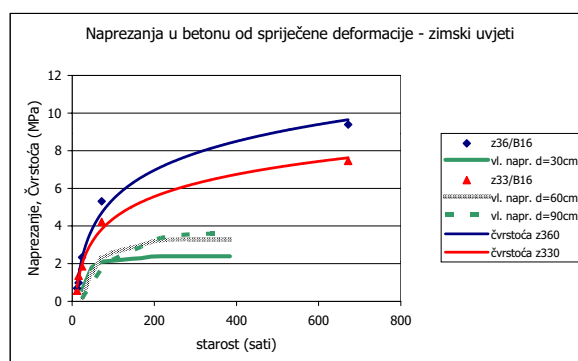
Slika 7. Prirast čvrstoće i naprezanja u betonu od spriječene deformacije za a) ljetne uvjete i b) zimske uvjete
