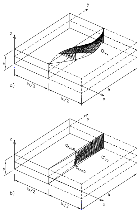
Slika 3. Normalna naprezanja u ravlini x = l_x/2 : a) \sigma_{xx} , b) \sigma_{zz}
