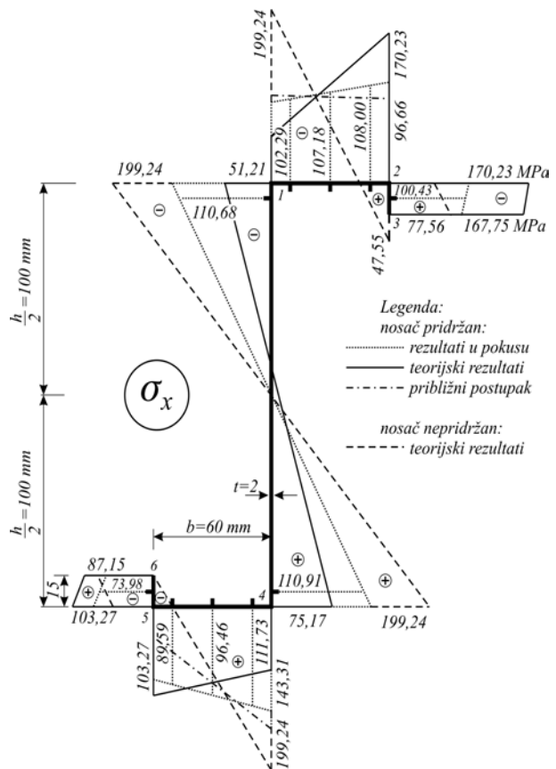
Slika 16. Model "A". Dijagrami normalnih napreznja u poprečnom presjeku u sredini raspona nosača
