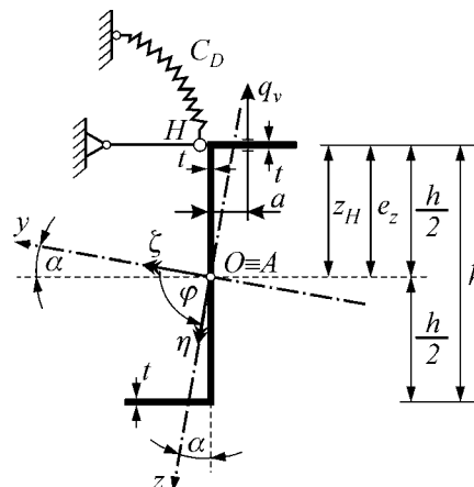
Slika 6. Bočno pridrzan tankostijeni nosač Z- profila pod djelovanjem odličućeg opterećenja
