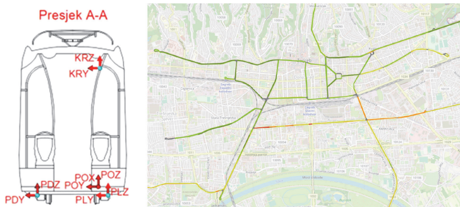
Slika 1. Prikaz pozicija akcelerometara na vozilu i izračunatih razina udobnosti vožnje na zagrebačkoj tramvajskoj mreži
