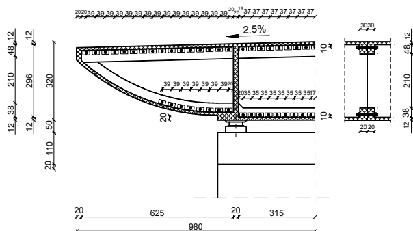
Slika 14. Raspored prednapetih šipki \phi 36 mm na spojevima odsječaka grede
