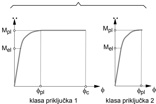
Slika 6. Klase duktilnosti priključka – klasifikacija po rotacijskom kapacitetu
