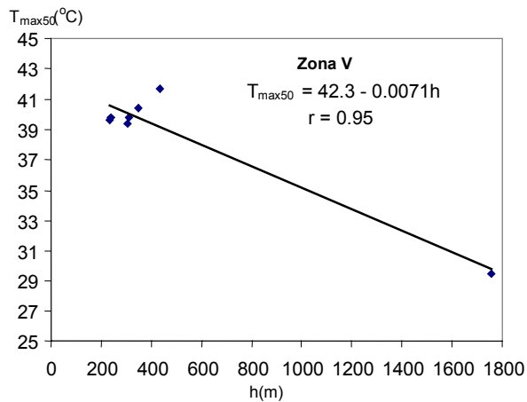
Slika 3. Vertikalni gradijenti najveće temperature zraka T_{max50} . Na ovoj je slici prikazano pet grafikona na kojima su nacrtani regresijski pravci koji su dobiveni interpolacijom vrijednosti odnosa između najvećih temperatura zraka koje se mogu očekivati jednom u 50 godina i nadmorske visine, za razdoblje 1961.-1990.
