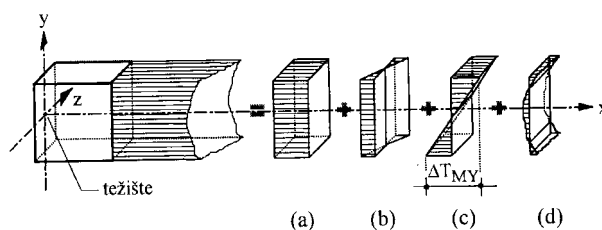
Slika 1. Raspodjela temperature prikazana sa 4 konstituiraјуće komponente
