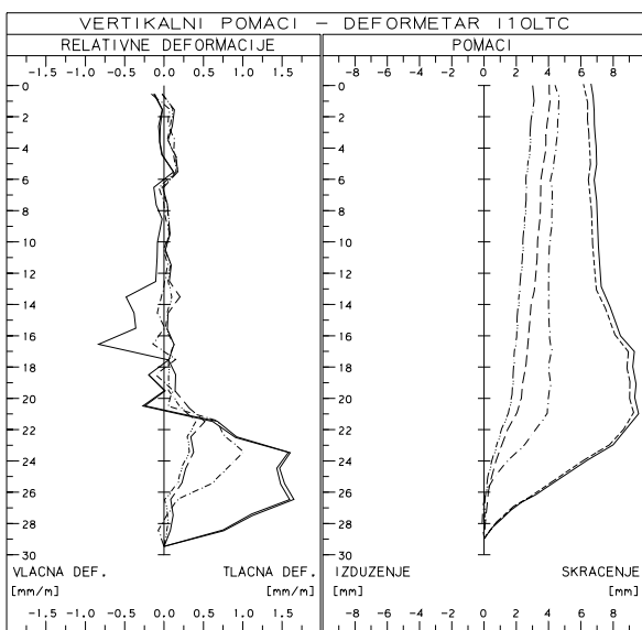
Slika 7. Vertikalni pomaci - deformetar I10LTC
