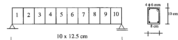
Slika 2. Armiranobetonska gredica
