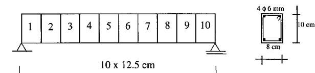
Slika 2. Armiranobetonska gredica
