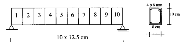
Slika 2. Armiranobetonska gredica
