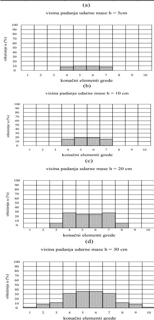
Slika 5. Dijagrami oštećenja gredica udarnim opterećenjem: a) h = 5 \text{ cm} , b) h = 10 \text{ cm} , c) h = 20 \text{ cm} , d) h = 30 \text{ cm}
