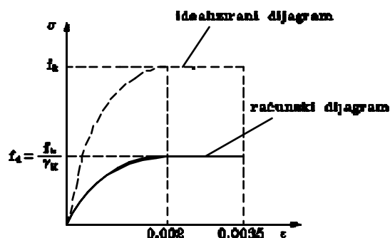
Slika 6. Računski dijagram naprezanja ( \sigma ) - relativna deformacija ( \varepsilon )
