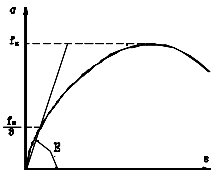
Slika 5. Dijagram naprezanja ( \sigma ) - relativna deformacija ( \varepsilon ) tlačno opterećenog zida
