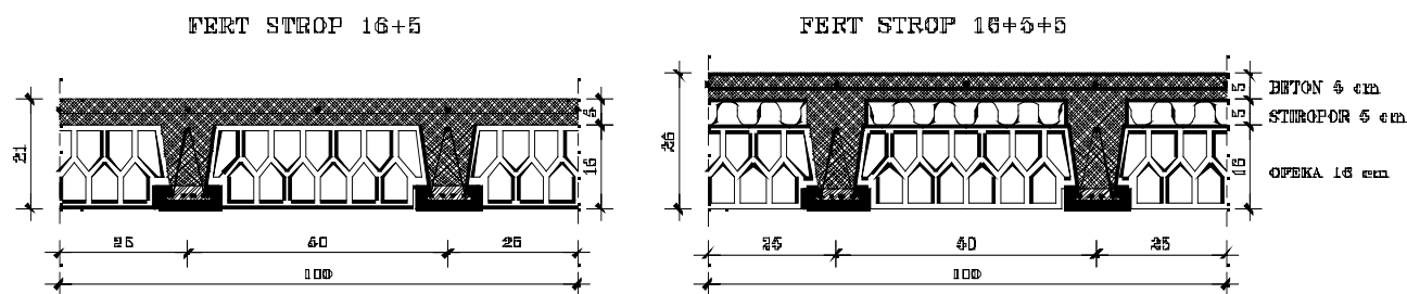
Slika 3 Poprečni presjeci fert-stropova F(16+5) i F(16+5+5)
