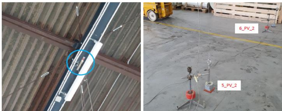
Slika 7.13 Pogled na sekundarni nosač br. 5 i susjedne nosače br. 4 i 6 sa označenim mjernim mjestima vertikalnih pomaka (oznaka PV), horizontalnog pomaka (oznaka PH) i relativnih deformacija (oznaka RD)
