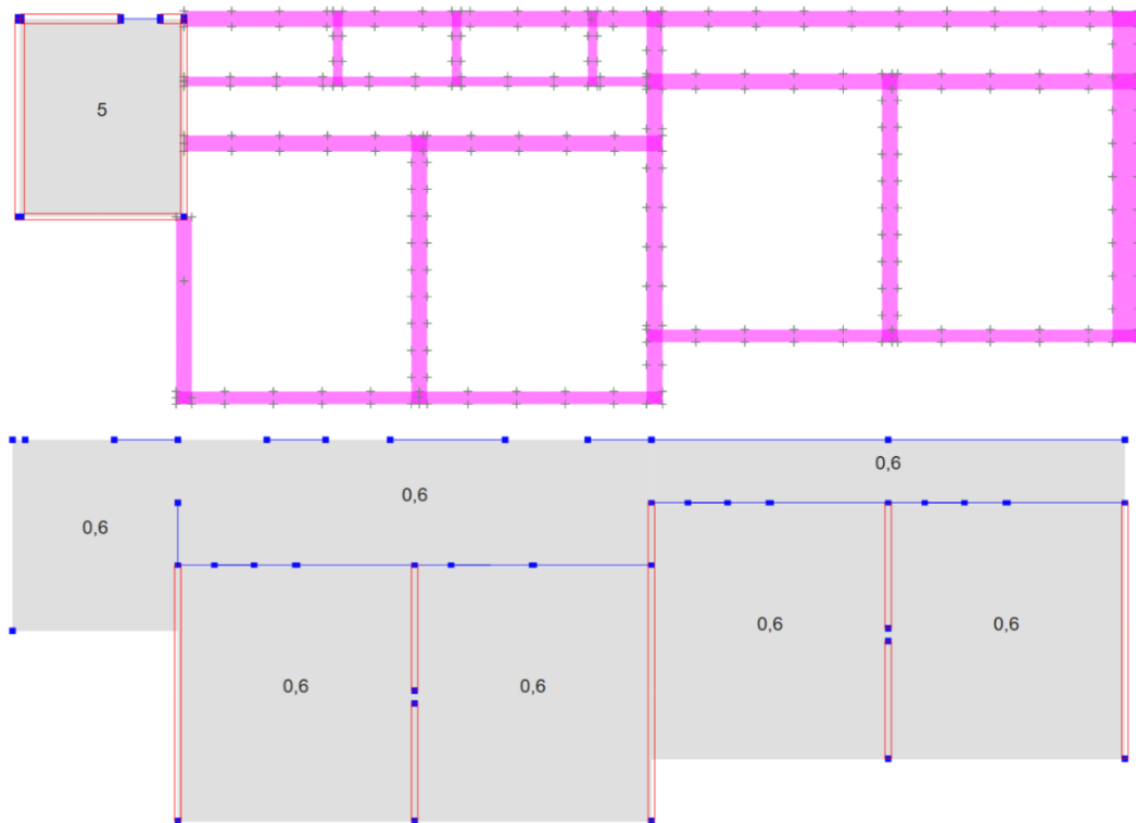
Slika 22: Shema korisnog opterećenja na stropnim pločama podruma (gore) i prizemlja (dolje) [ \text{kN/m}^2 ]
