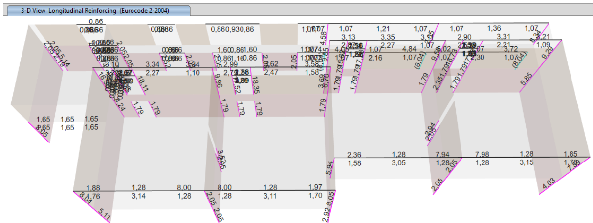
Slika 168: Potrebne količine uzdužne armature u stupovima i horizontalnim serklažima prema mjerodavnoj kombinaciji PTRRSQ [cm 2 ]
