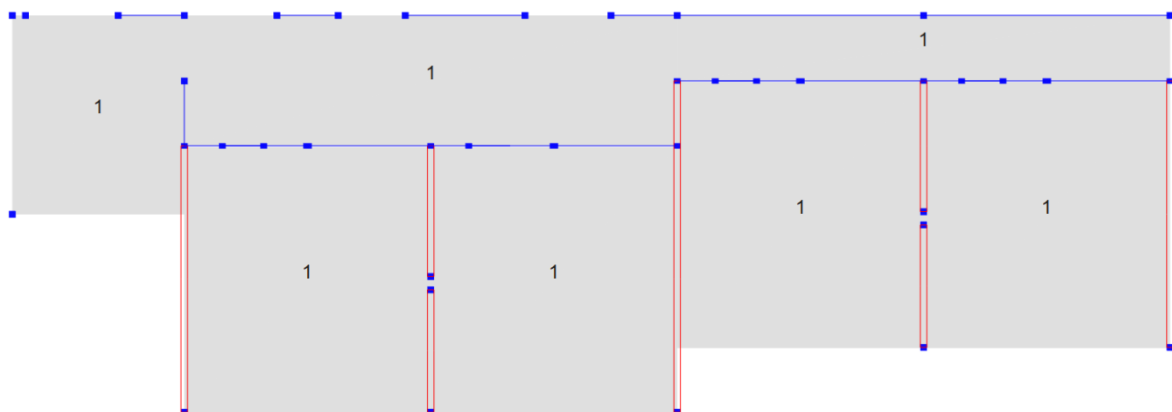
Slika 23: Shema opterećenja snijegom na stropnoj ploči prizemlja [ \text{kN/m}^2 ]
