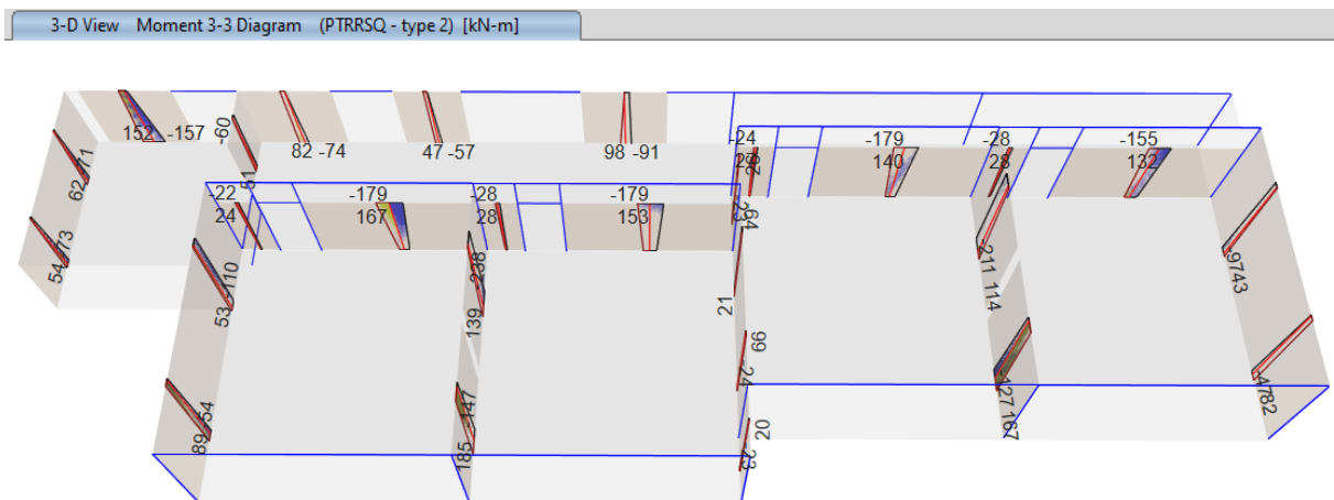
Slika 138: Raspodjela momenata savijanja integriranih po dužini zida kata od mjerodavne kombinacije PTRRSQ [kNm]
