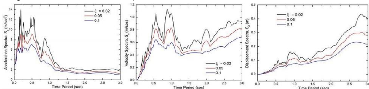
a.)spektar ubrzanja
