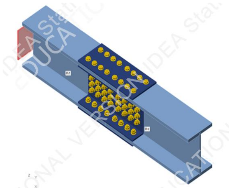
Slika 10.45. Prikaz priključka
