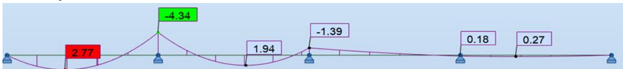
Slika 10.23. Maksimalan negativni moment savijanja
