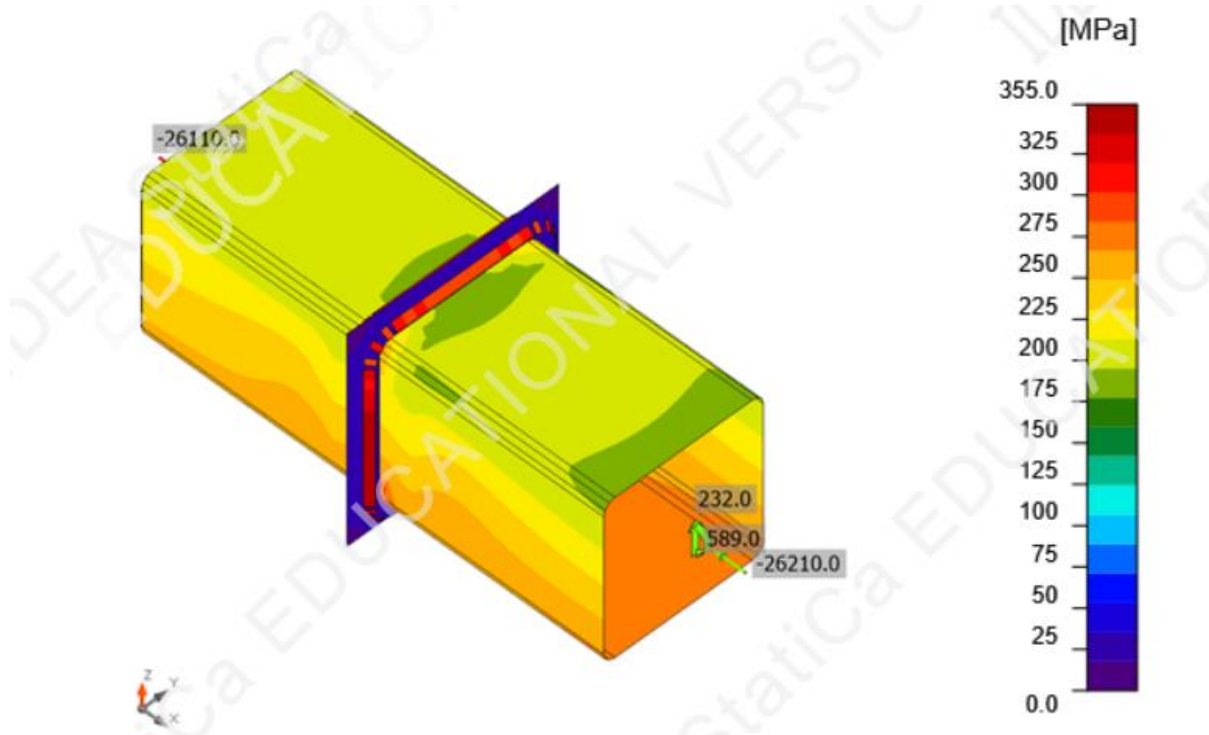
Slika 10.50. Raspodjela naprezanja priključka
