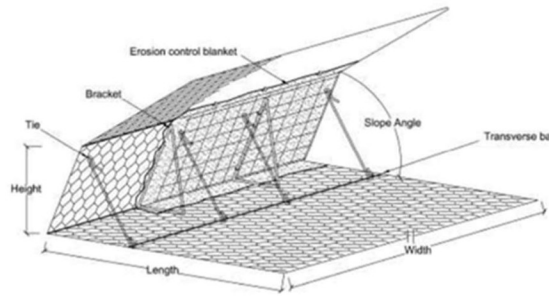
Slika 25. Shematski prikaz GREEN TERRAMESH sustava
