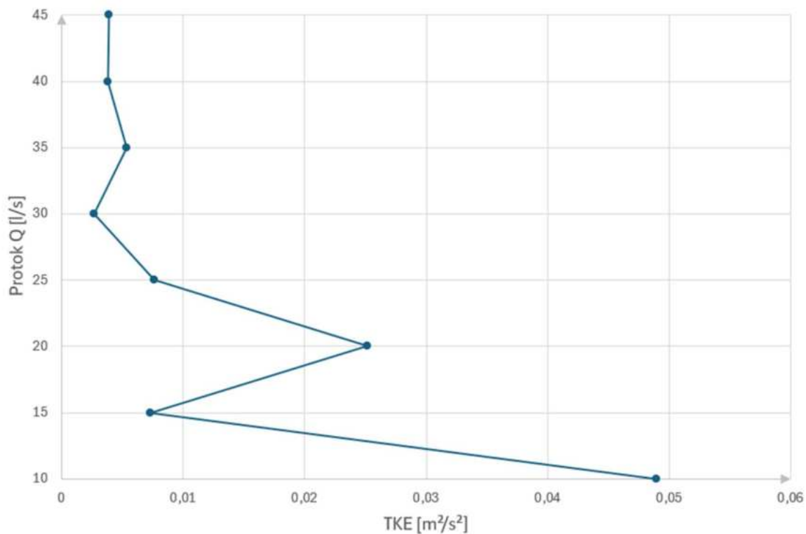
Slika 15. Grafički prikaz srednje turbulentne kinetičke energije po protocima Q
