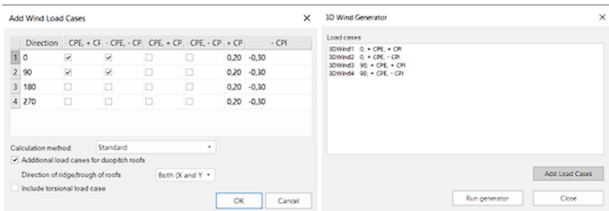
Slika 21.: Prikaz zadavanja parametara u programu SCIA Engineer
