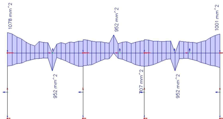
Slika 125.: Prikaz potrebne armature greda za X smjer – najniža cijev
