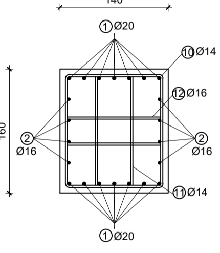
PRESJEK C-C MJ 1:25
