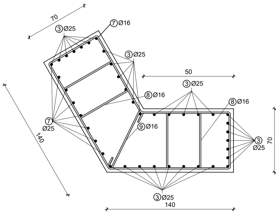
PRESJEK A-A MJ 1:25
