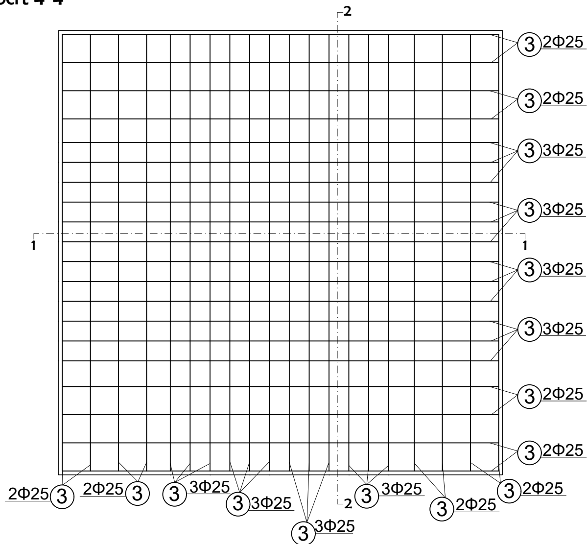
Tlocrt 4-4
