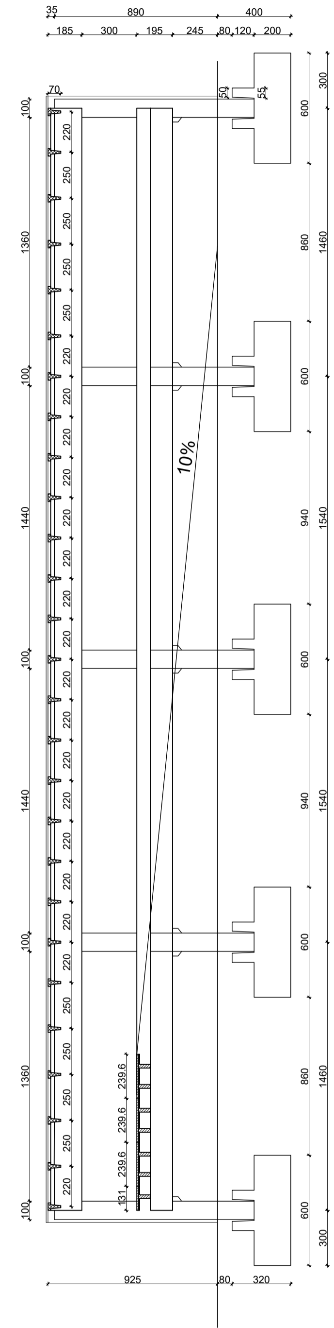
PRESIEK A-A
