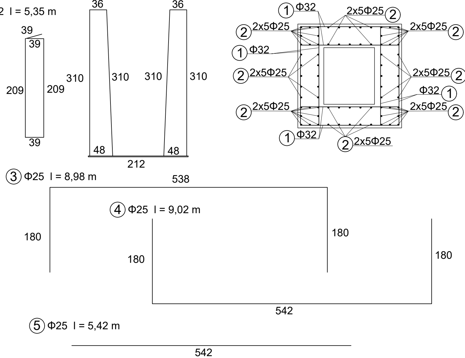
Tlocrt 3-3
