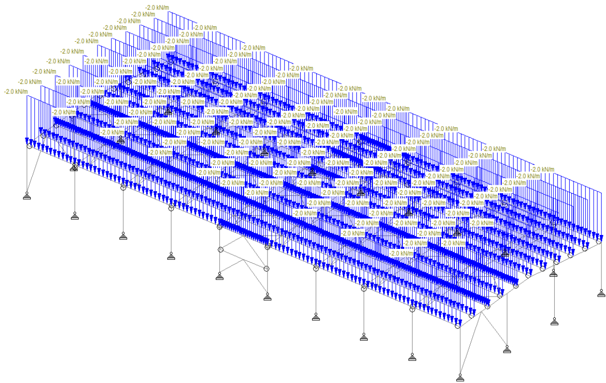
Slika 31: Opterećenje 2 – snijeg
