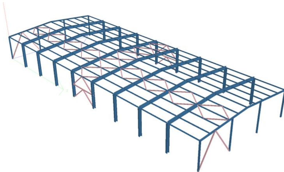
Slika 1: prostorni prikaz konstrukcije tip 1
