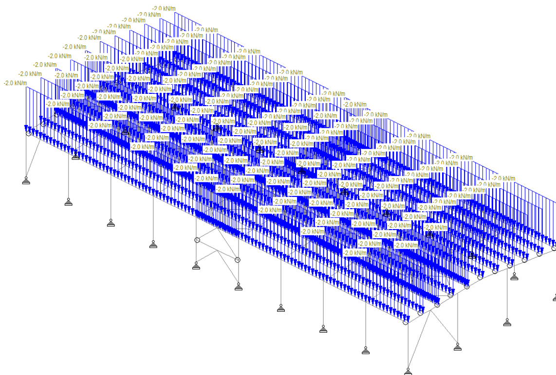
Slika 21: Opterećenje 2 – snijeg
