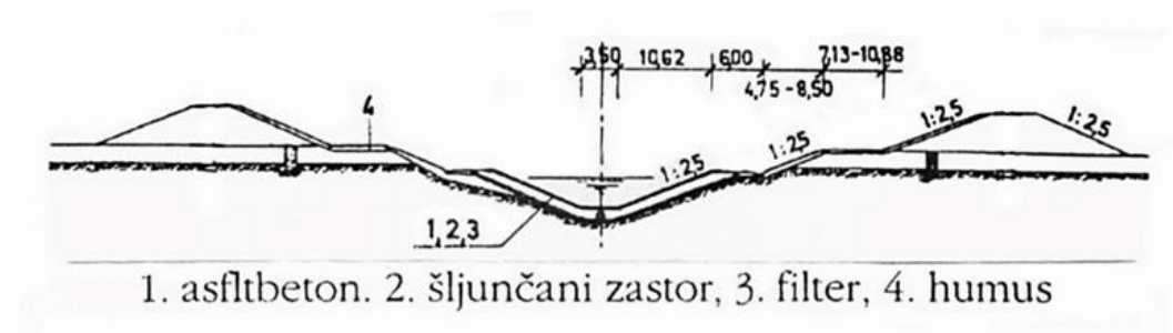
Slika 7. Asfaltbetonska obloga [2]
