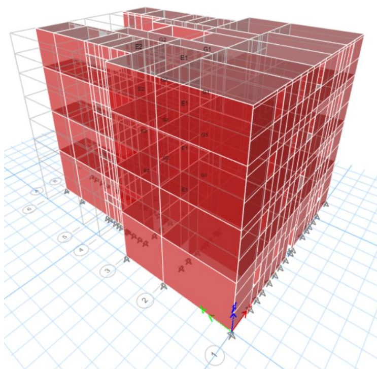
Slika 5. – model konstrukcije
