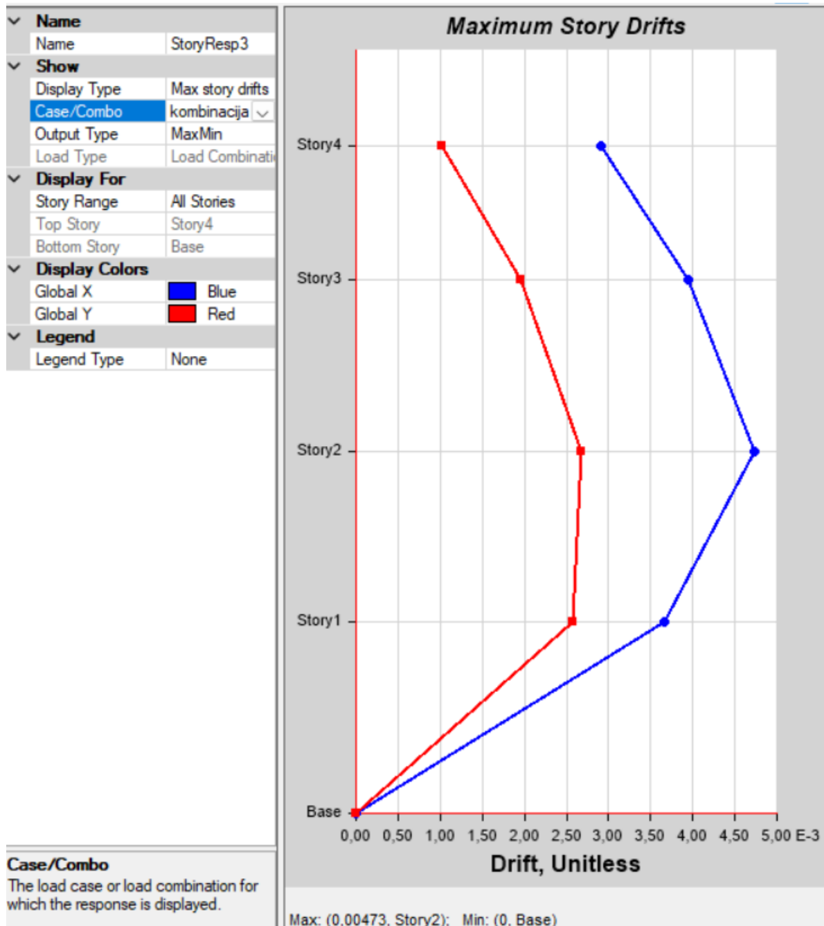
Slika 22. – maksimalni međukatni pomak
