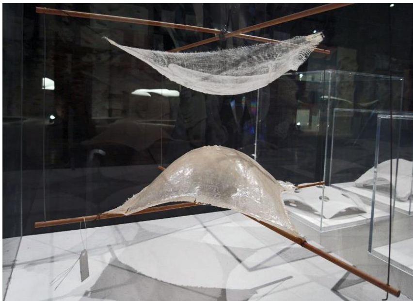
Slika 23.: Islerov viseći model (Izvor: [29])
