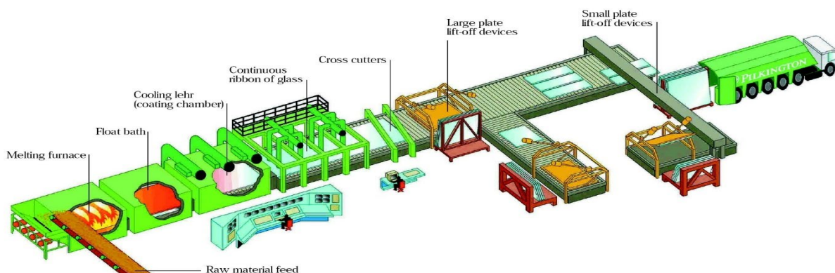
Slika 21.: Prikaz Pilkingtonovog procesa [17]
