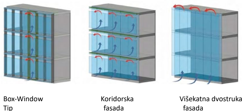
Slika 19.: Podjela dvostruko staklenih fasada [13]
