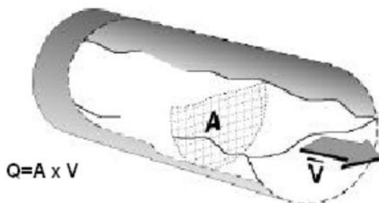
Slika 33: Skica otvorenog kanala i veličina (Izvor:[8])
