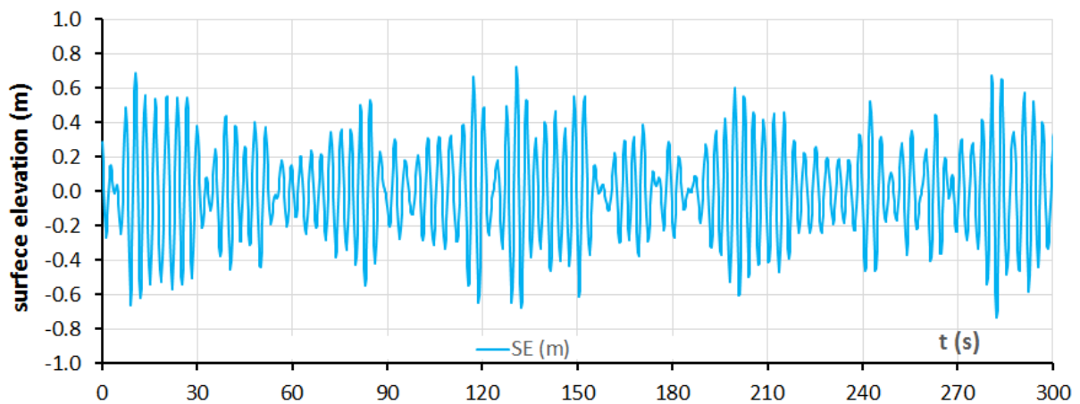
Slika 2.5 Karakteristična sekvenca dinamike morskih razi na liniji generiranja (JONSWAP spektar ; \gamma = 3,3 ; H_s=1,0\text{m} ; T_p =3,3\text{s} ; direkcionalna disperzija 30^0 )
