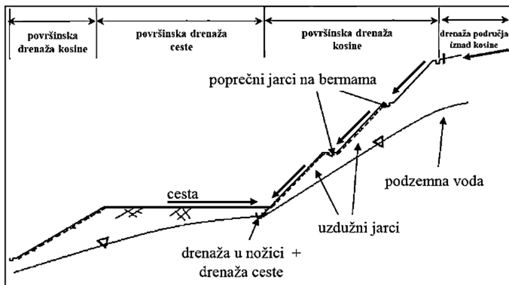
Slika 2.: Površinska drenaža uz ceste (Izvor: [1])
