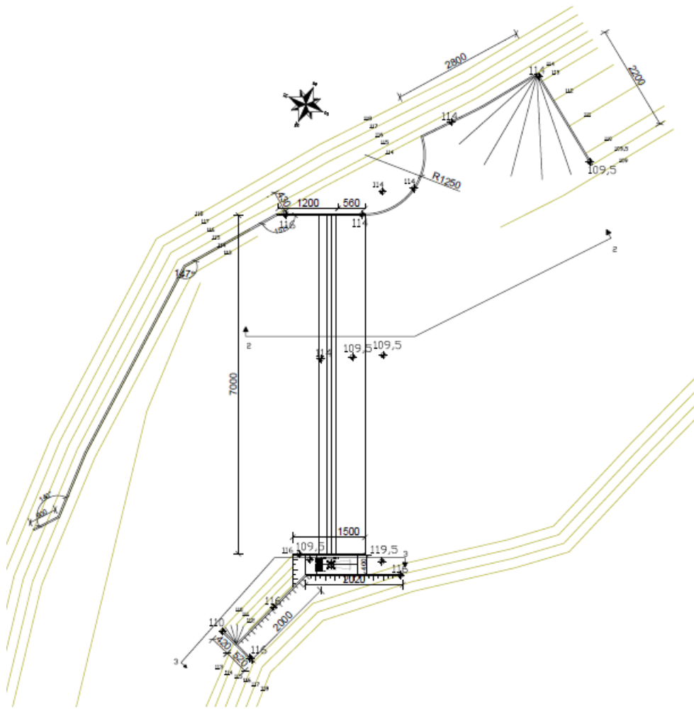
Slika 19 Tlocrt varijante 3
