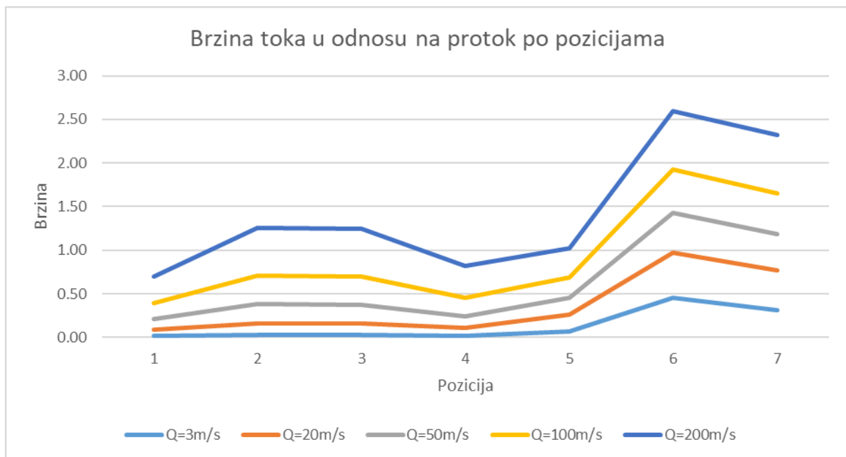
Slika 30 usporedba brzine tečenja u odnosu na protok po pozicijama za varijantu 1
