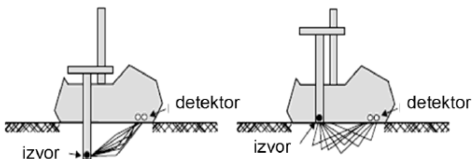
Slika 43. Nuklearni densimetar [7]
