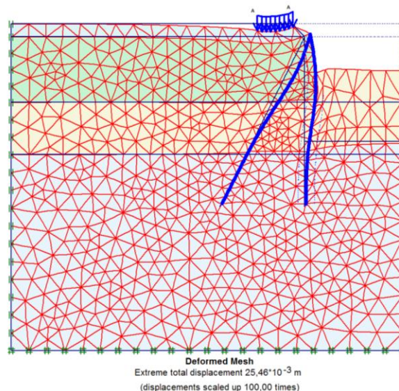
Slika 27. Deformabilnost modela u drugoj fazi
