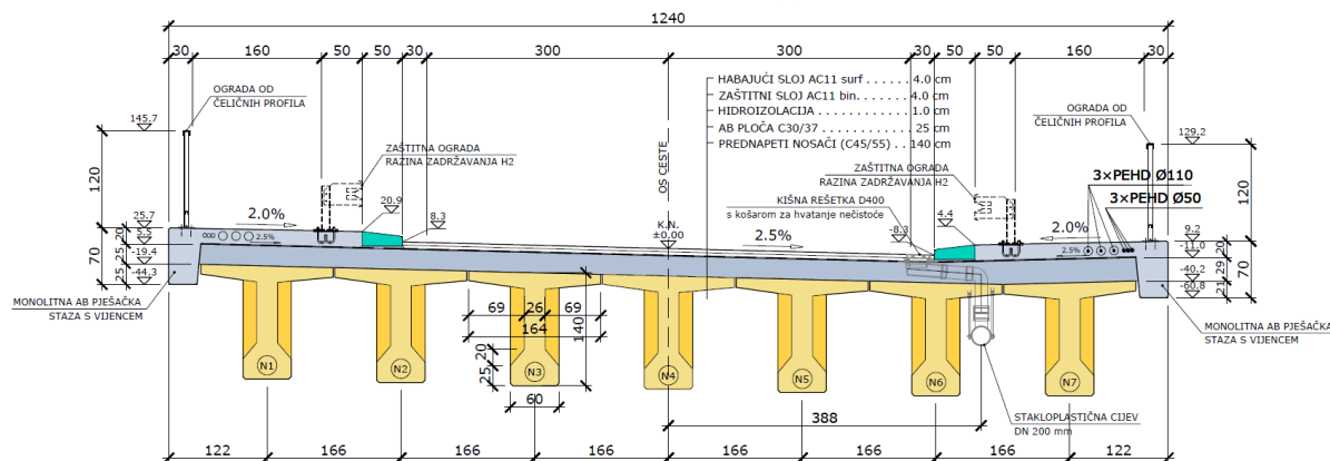
Slika 4. Nadvožnjak „Pavučnjak“, poprečni presjek [3]
