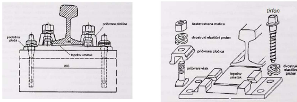
Pričvrсни pribor tipa K (njemački sistem) - 24 kg čelika po pragu
